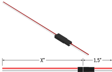
Power Connector (20/2 Gauge Wire) LLED8400-PC (33" Standard) LLED8400-PC-X (X = Specify Length)
